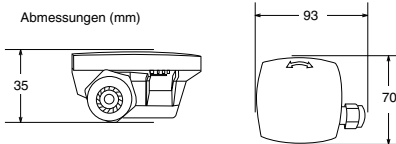
Abmessungen (mm)
