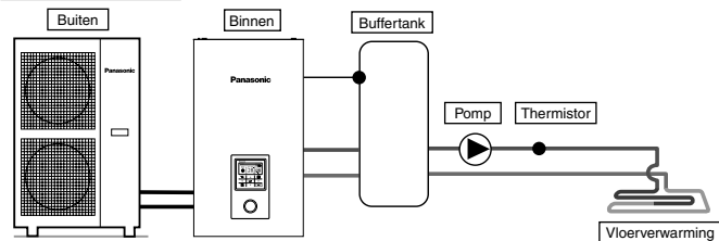
Aansluiting buffertank
