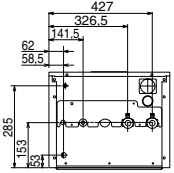
ALTINDAN GÖRÜNÜM
