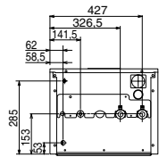
ΚΑΤΩ ΟΨΗ
