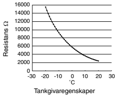
Tankgivaresistans i förhållande till temperatur
