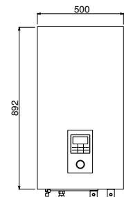
ΜΠΡΟΣΤΙΝΗ ΟΨΗ
