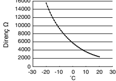
Tank sensörü karakteristik özellikleri
