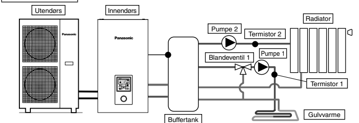
Gulvvarme + radiator
