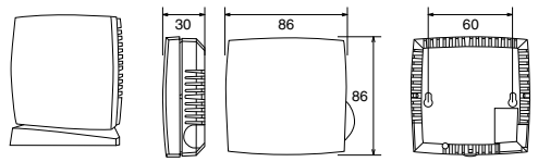
Abmessungen (mm)
