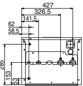
ΚΑΤΩ ΟΨΗ
