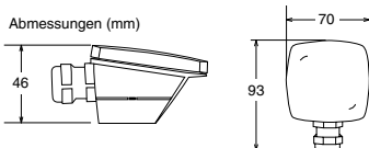
Abmessungen (mm)
